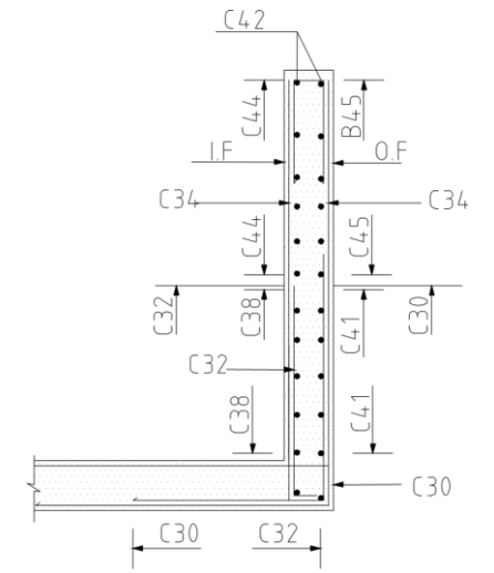
SECTION D - D. 1:25
