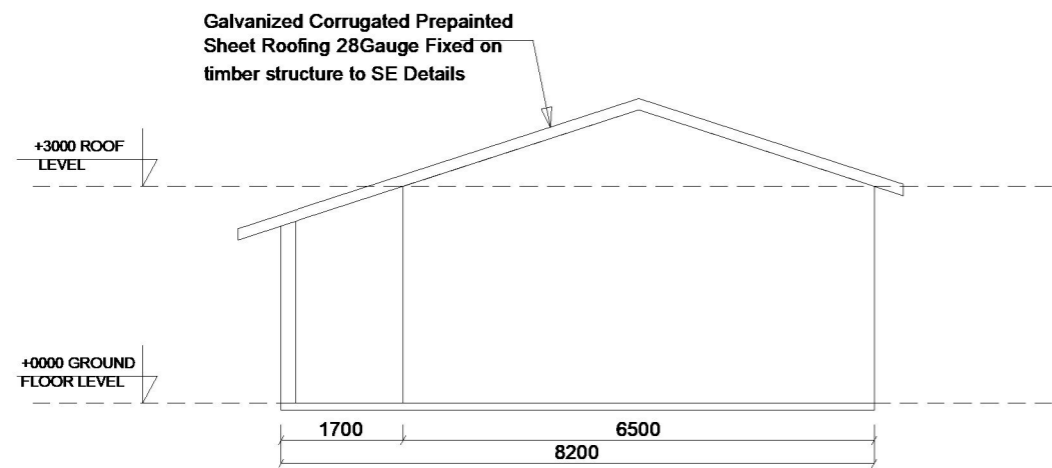
ELEVATION 02
