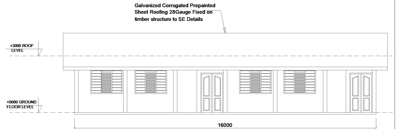
ELEVATION 01
