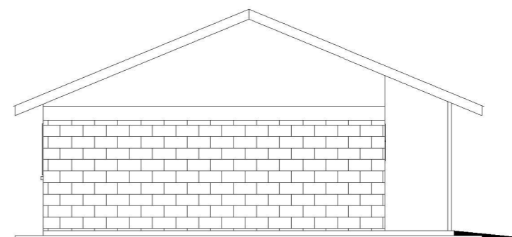
ELEVATION 04
