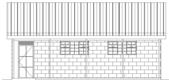
ELEVATION 01
