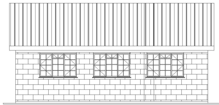
ELEVATION 02
