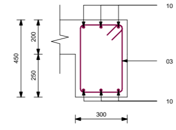
Section 3-3 1 : 10
