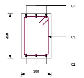
RB2 Section 7-7 1 : 10
