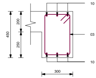
TB2 Section 2-2 1 : 10
