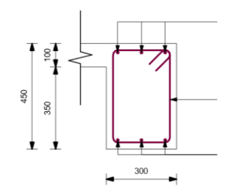
GB2 Section 8-8 1 : 10
