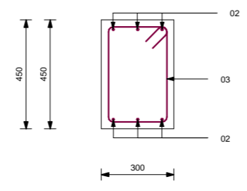
RB1 Section 5-5 1 : 10
