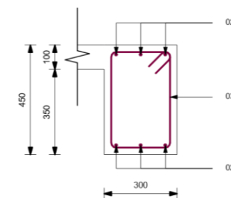
GB2 Section 7-7 1 : 10
