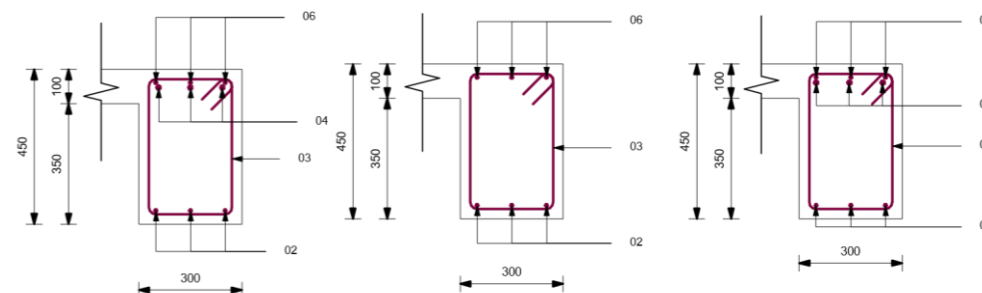
GB1 Section 3-3 1 : 10
