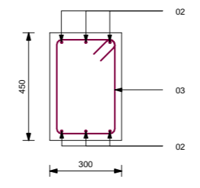
RB2 Section 8-8 1 : 10
