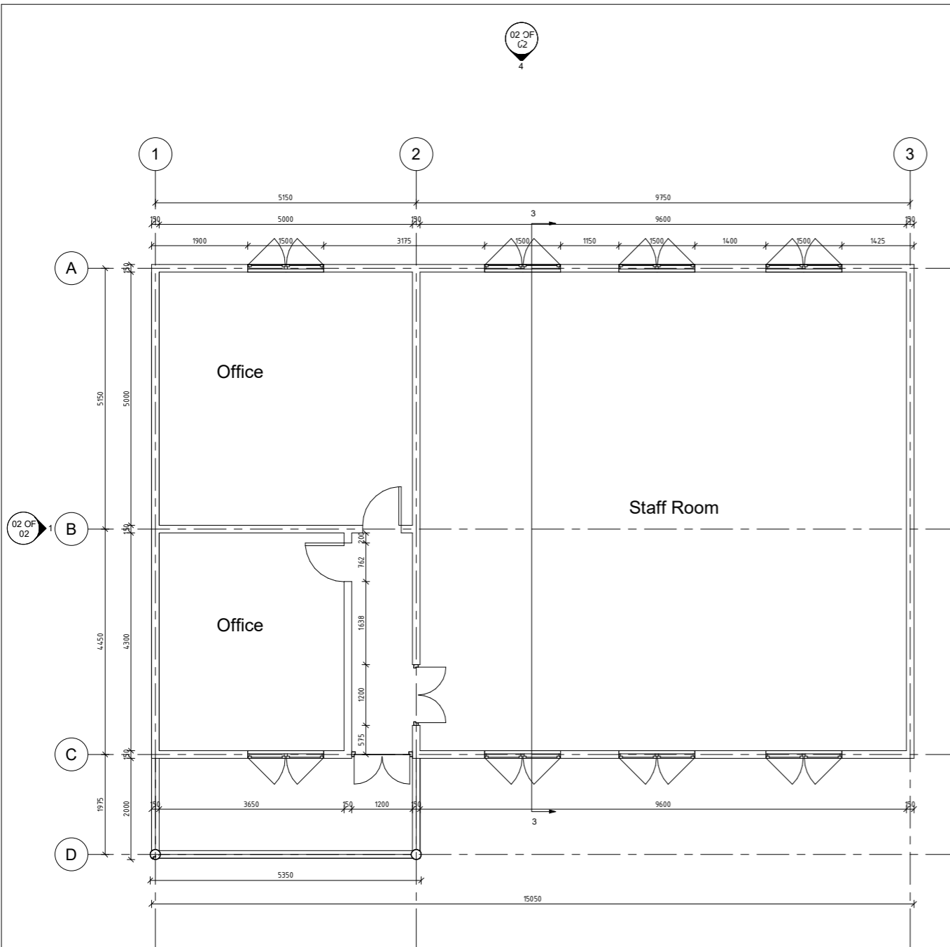
1 FLOOR PLAN 1 : 50
