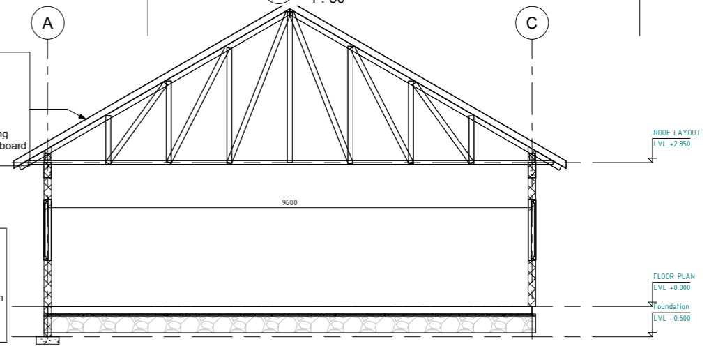
3 section 3-3 1 : 50
