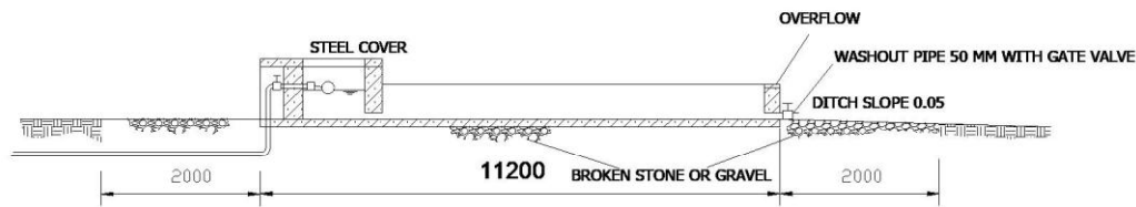
SECTION A-A
